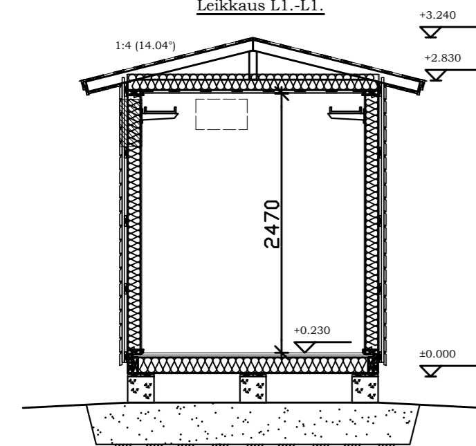
Leikkaus L1.-L1.
